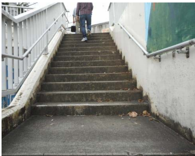
上倉田町 464 付近 階段の劣化状況（左）と隧道照明器具⑧の故障状況（右）（10月21日 撮影）
